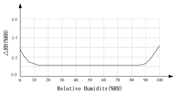
图 2: 25℃时 AM2305 的相对湿度最大误差
