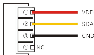
图 1：AM2305 引脚分配图
